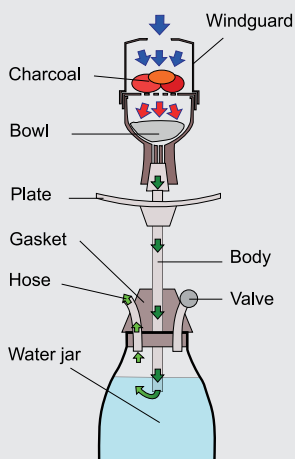
Рисунок 1. Компоненты кальяна
