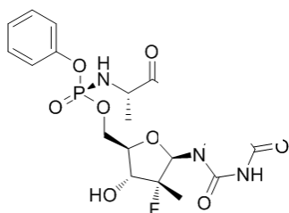
Sofosbuvir
